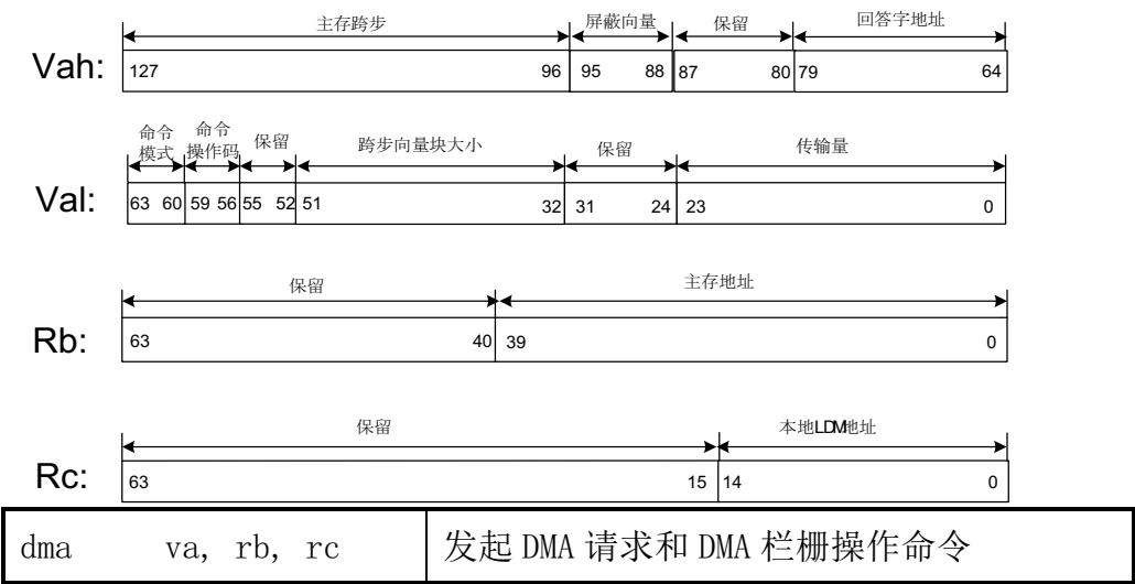
图 5-1 DMA 参数各字段功能
