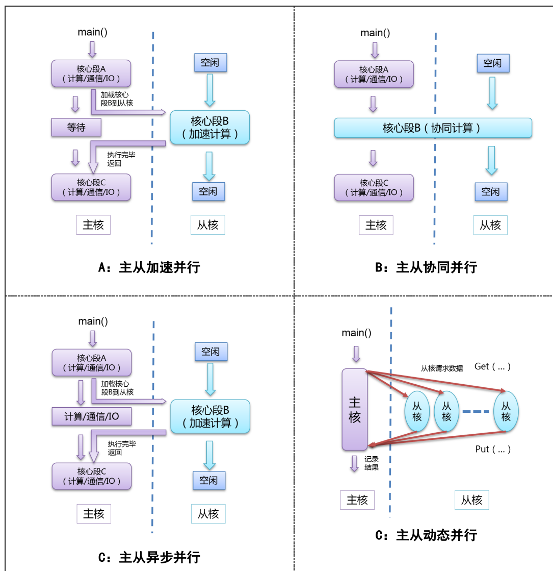
图 1-6 “神威太湖之光”计算机系统异构并行方法
