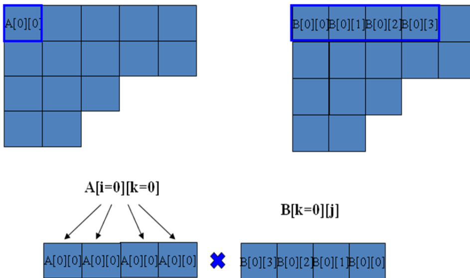
图 5-10 矩阵乘向量化优化示例
