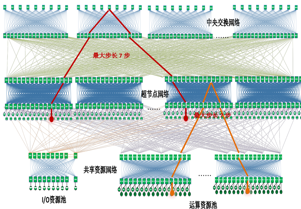
图 1-4 高速计算互连网络拓扑连接示意图
