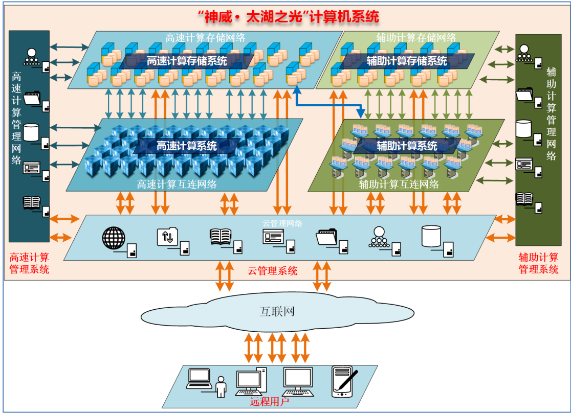
图 1-1 “神威·太湖之光”系统总体架构图
