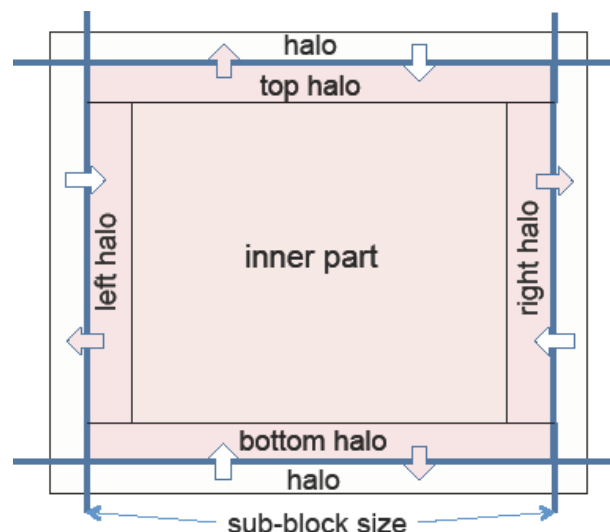
图 9-11 面向计算通信重叠的 sub-block 划分
