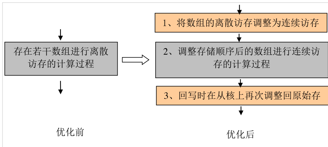
图 5-7 离散访存问题的优化示意图
