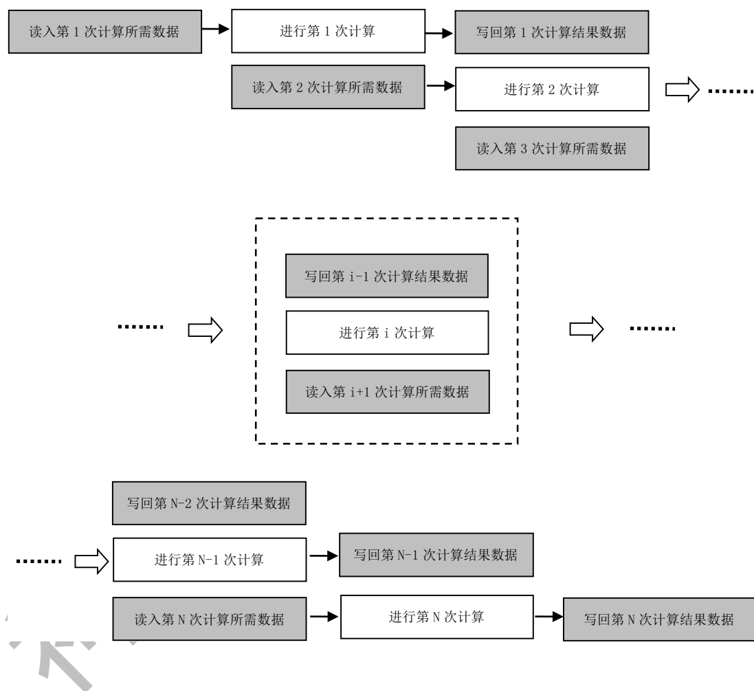
图 9-6 双缓冲机制下通信和计算互相隐藏原理示意图
