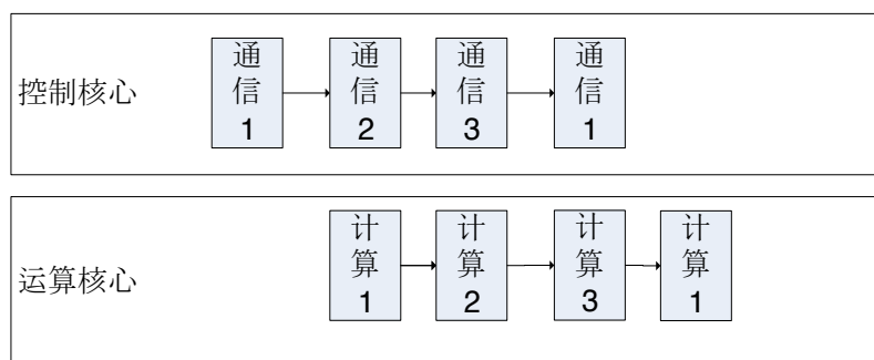
图 7-2 通信隐藏算法
