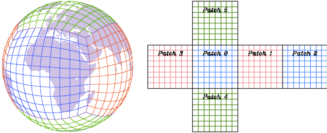
图 9-7 球立方网格系统
