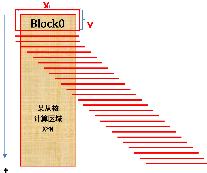
图 9-13 Inner Part 运算核心计算方案
