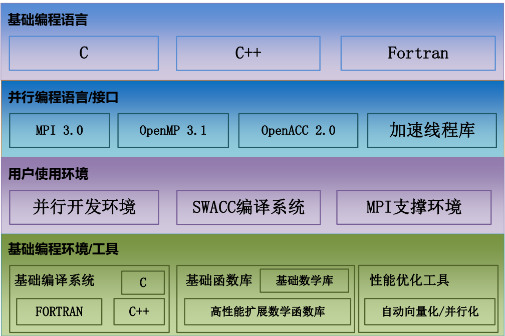
图 1-5 “神威太湖之光”计算机系统语言环境组成结构图
