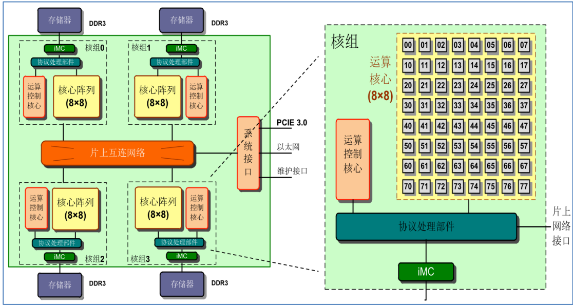
图 1-2 “申威 26010” 异构众核处理器架构图
