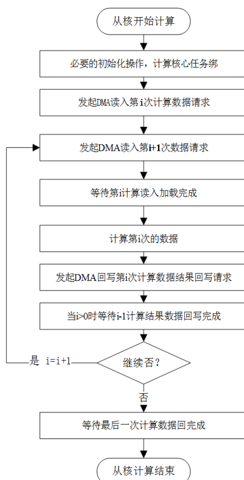
图 9-5 从核心双缓冲机制示意图
