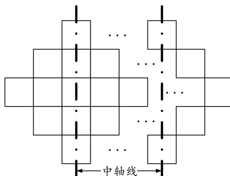
图 9-14 Stencil 对齐情况示意
